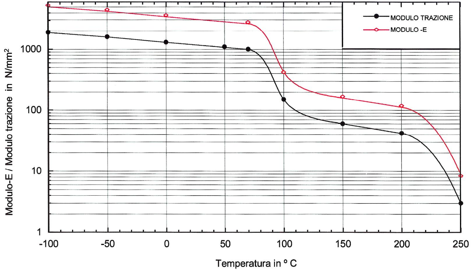
ZX100K: MODULO-E / MODULO TRAZIONE ESPRESSO IN f ( TEMPERATURA °C)
